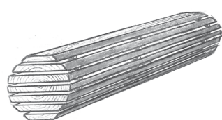
Plots
